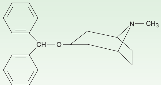
Benztropine
