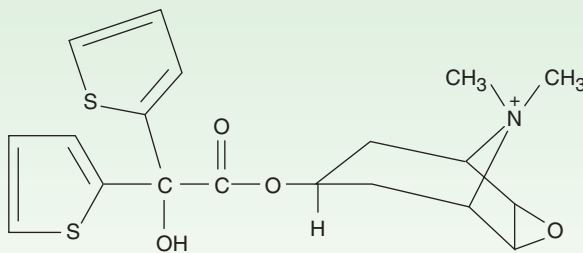
Tiotropium
